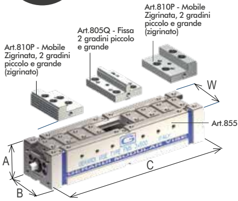
Art.864 Morsa doppia singola autocentrante con ganasce a doppio gradino zigrinate. Disponibile A RICHIESTA con ganasce lisce (8100)
